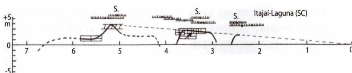
Figura 21. Oscilações do nível relativo do mar nos últimos 7.000 anos, segundo SUGUIO (2005). Obs.: O gráfico identifica a dinâmica do nível marinho para o trecho Itajaí-Laguna.
