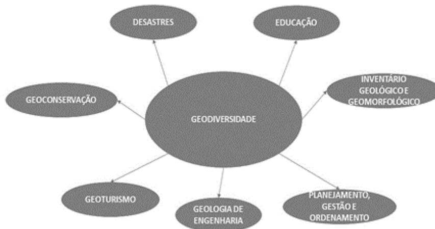
Figura 02. Geodiversidade. Adaptado de CPRM (2008)
